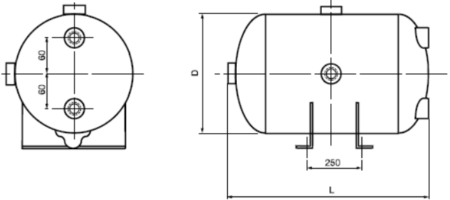
5 Ports M22x1,5
