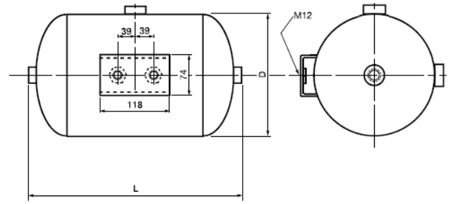
4 Ports M22x1,5
