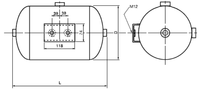
4 Ports M22x1,5
